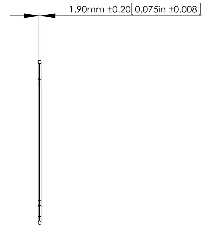
SECTION A-A SCALE 2 : 3
