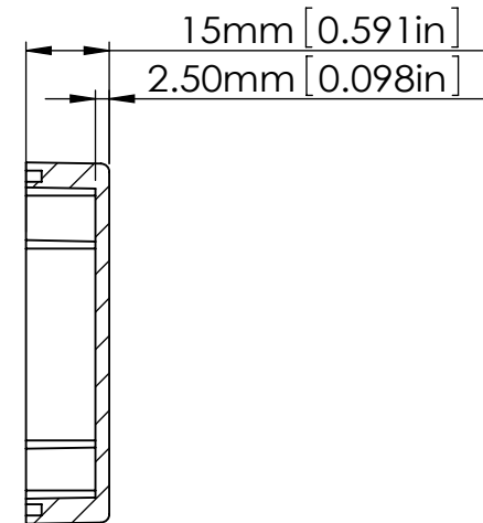
SECTION B-B SCALE 2 : 3
